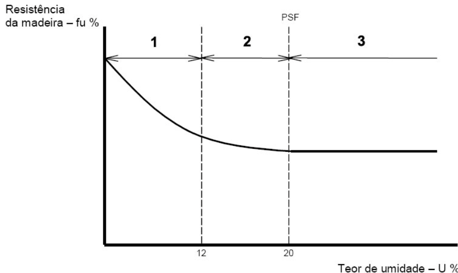
Figura 1: Gráfico resistência da madeira x teor de umidade (ALMEIDA, 1998).
